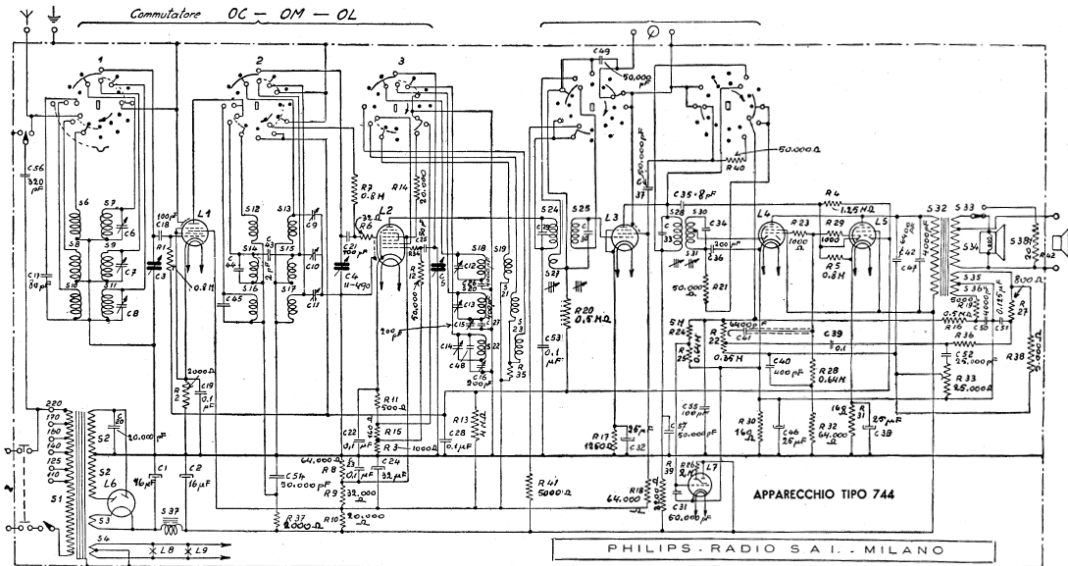
105. — PHILIPS RADIO — Mod. 744. — Produzione 1939-1940. — Media frequenza: 468 kHz. — Gamme: c. c. (16-32 m), c. (28-501 m), m. (180-580 m), l. 700-2000 m.). — Sintonizzazione automatica per 8 stazioni. — Selettività variabile da 8 a 15 kHz. — Valvole: L1 = EF8, L2 = EK2, L3 = EF9, L4 = EBL1, L5 = EBL1, L6 = WE53, L7 = EM1.
